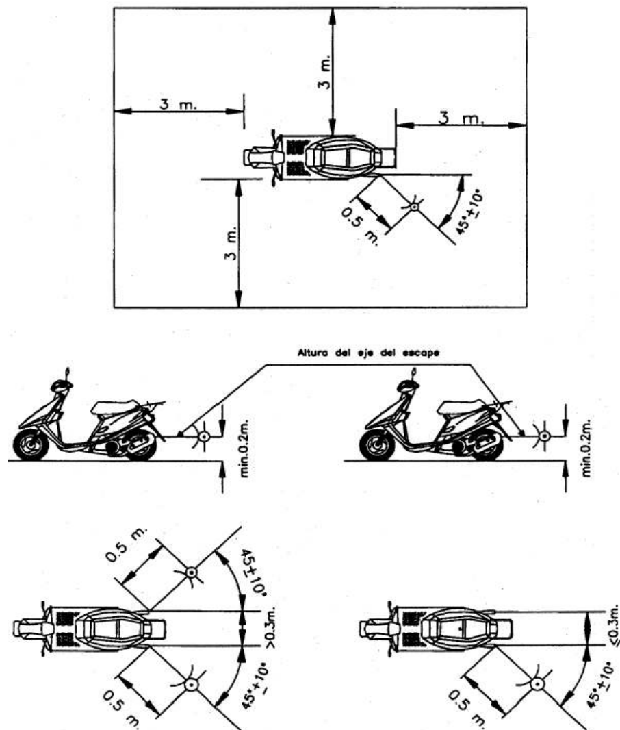
Figura 1. Posiciones para el ensayo de las motocicletas paradas
